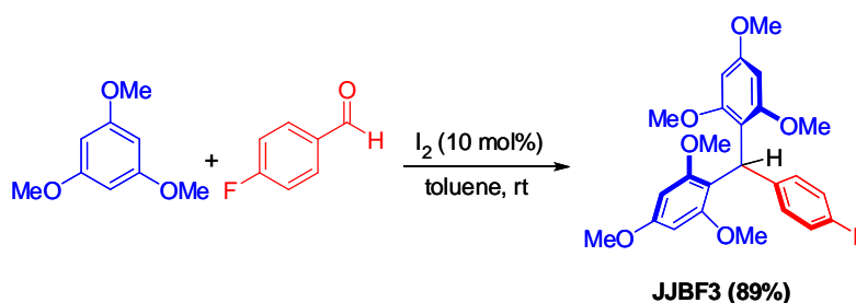
รูปที่ 28 การสังเคราะห์สาร fluorinated triarylmethanes (JJB3)
