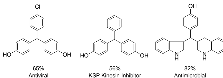
รูปที่ 12 ปฏิกริยาการสังเคราะห์ triarylmethane ที่มีฤทธิ์ทางชีวภาพโดยใช้ตัวเร่งปฏิกิริยาผสมระหว่าง [\text{Ir}(\text{COD})\text{Cl}]_2 กับ \text{SnCl}_4
