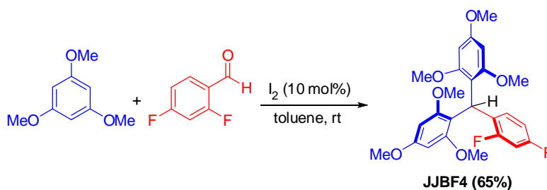
รูปที่ 29 การสังเคราะห์สาร fluorinated triarylmethanes (JJBF4)
