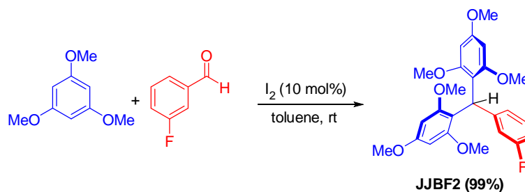
รูปที่ 27 การสังเคราะห์สาร fluorinated triarylmethanes (JJB2)
