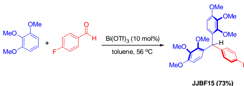
รูปที่ 38 การสังเคราะห์สาร fluorinated triarylmethanes (JJBF15)
