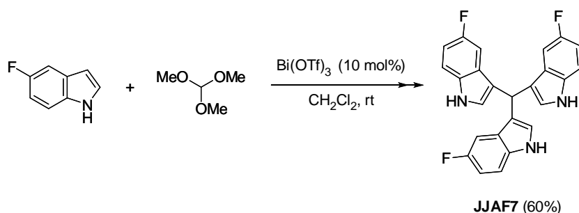
รูปที่ 25 การสังเคราะห์สาร fluorinated triarylmethanes (JJAF7)
