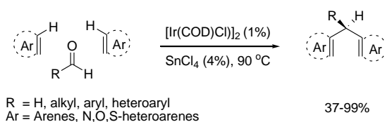
รูปที่ 11 ปฏิกริยาการสังเคราะห์ triarylmethane และ diarylalkylmethane โดยใช้ตัวเร่งปฏิกิริยาผสมระหว่าง [\text{Ir}(\text{COD})\text{Cl}]_2 กับ \text{SnCl}_4
