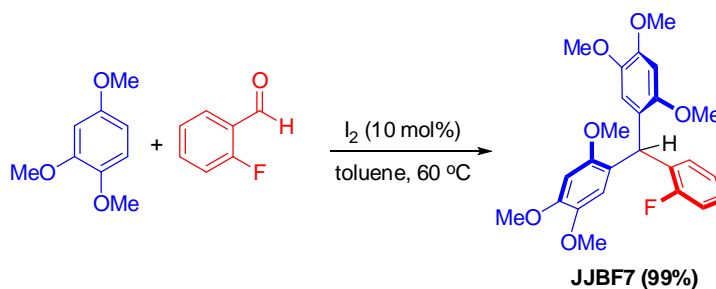
รูปที่ 32 การสังเคราะห์สาร fluorinated triarylmethanes (JJB7)
