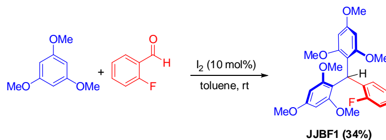
รูปที่ 26 การสังเคราะห์สาร fluorinated triarylmethanes (JJB1)
