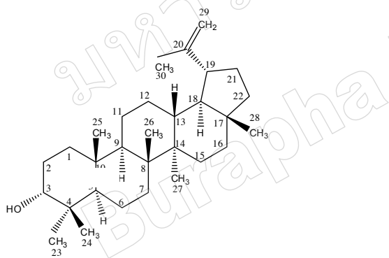
ภาพที่ 1 สูตรโครงสร้างของ Lupeol
