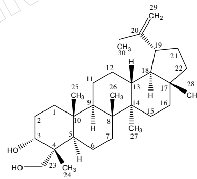
ภาพที่ 2 สูตรโครงสร้างของ lup-20(29)-ene-3 \alpha , 23-diol
