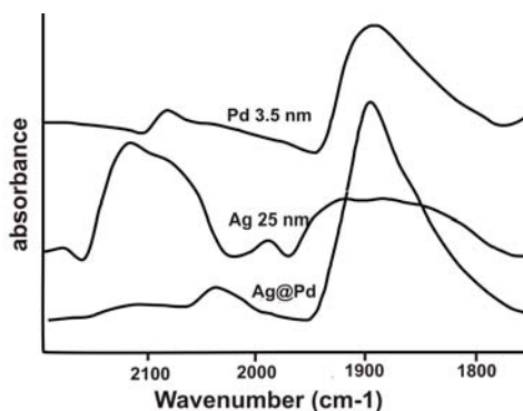
ภาพที่ 4 อินฟราเรดสเปกตรัมของ CO ดูดซับบนอนุภาคนาโนโลหะ แพลเลเดียม และโลหะเงิน@แพลเลเดียม อัตราส่วนโดยโมล 1:1
