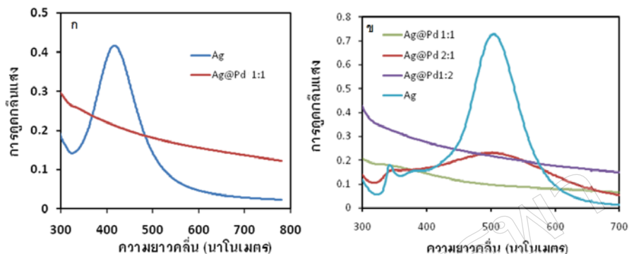
ภาพที่ 3 พลาสมอนเรโซแนนซ์สเปกตรัม ก) อนุภาคนาโนโลหะเงินรูปทรงกลม และอนุภาคนาโนโลหะเงิน@แพลเลเดียมรูปทรงกลม อัตราส่วน 1:1 ข) อนุภาคนาโนโลหะรูปแผ่น และอนุภาคนาโนโลหะคู่เงิน@แพลเลเดียมรูปแผ่น ที่อัตราส่วนจำนวนโมลเงินต่อแพลเลเดียมต่างๆ กัน
