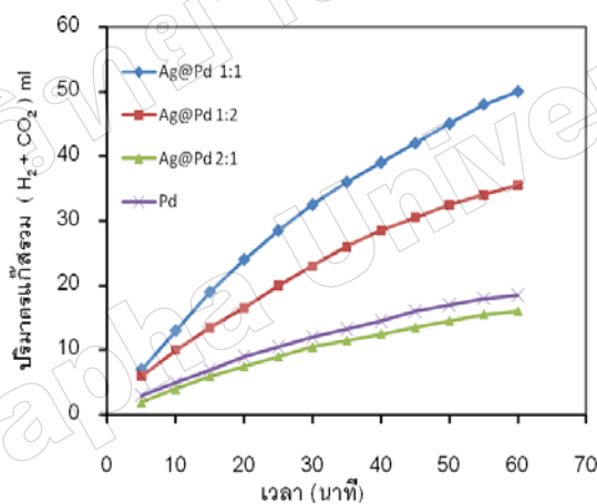
ภาพที่ 5 ปริมาตรแก๊สรวม ( \text{H}_2 และ \text{CO}_2 ) จากปฏิกิริยาการสลายตัวของกรดฟอร์มิกที่อุณหภูมิห้อง 30 องศาเซลเซียส โดยใช้ ตัวเร่งปฏิกิริยานาโนโลหะเงิน@แพลเลเดียมรูปแบบ (ปริมาณตัวเร่งปฏิกิริยาที่ใช้เท่ากับ 0.008 กรัม)
